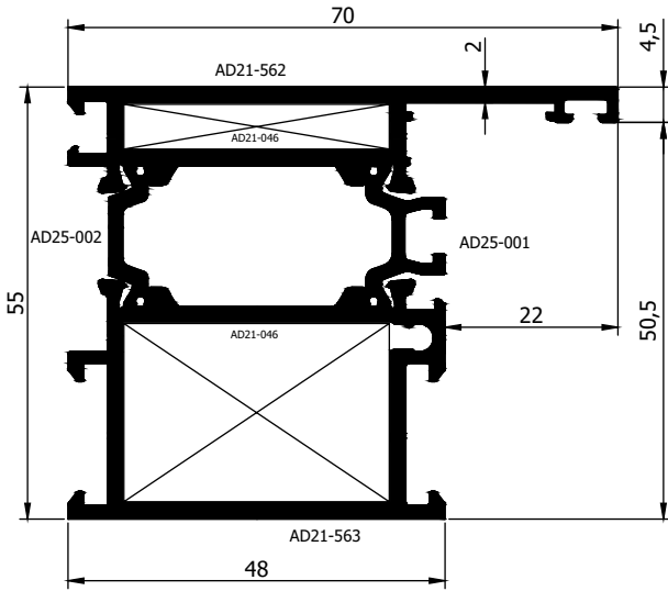
AD 21 - 051 ( 1,768 Kg/m )
