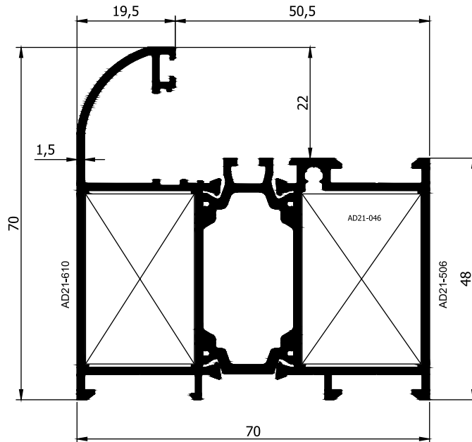
AD 21 - 088 ( 1,648 Kg/m )
