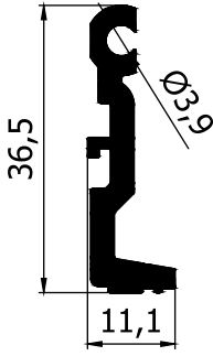
ORTA KAYIT BAĞLANTI PROFİLİ AD21-076 (0,420 Kg/m)
