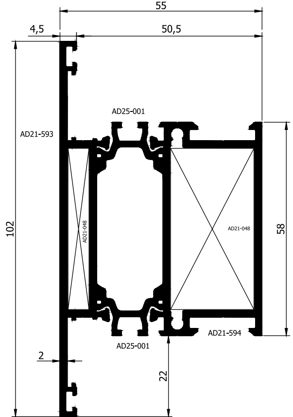
AD 21 - 068 ( 2,146 Kg/m )
