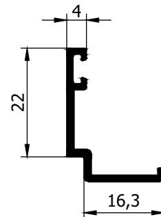
AD 20 - 040 ( 0,200 Kg/m )
