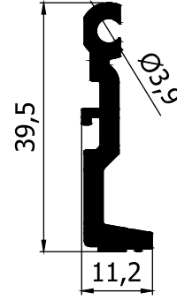
ORTA KAYIT BAĞLANTI PROFİLİ AD21-075 (0,444 Kg/m)
