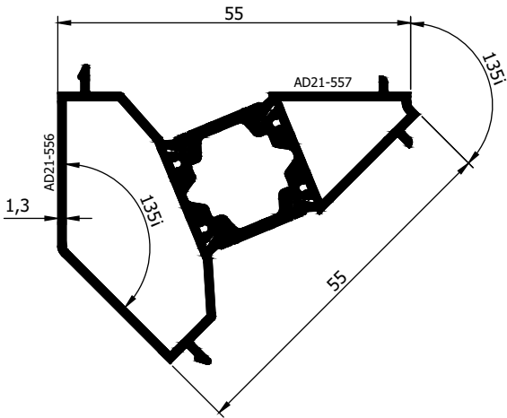
AD 21 - 031 ( 0,900 Kg/m )
