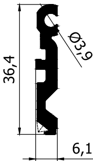
ORTA KAYIT BAĞLANTI PROFİLİ (SETSKURLU) AD21-077 (0,388 Kg/m)
