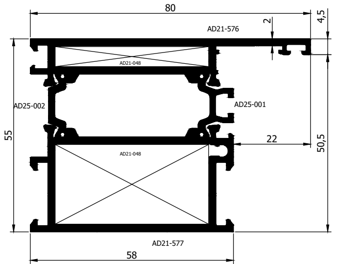
AD 21 - 058 ( 1,980 Kg/m )
