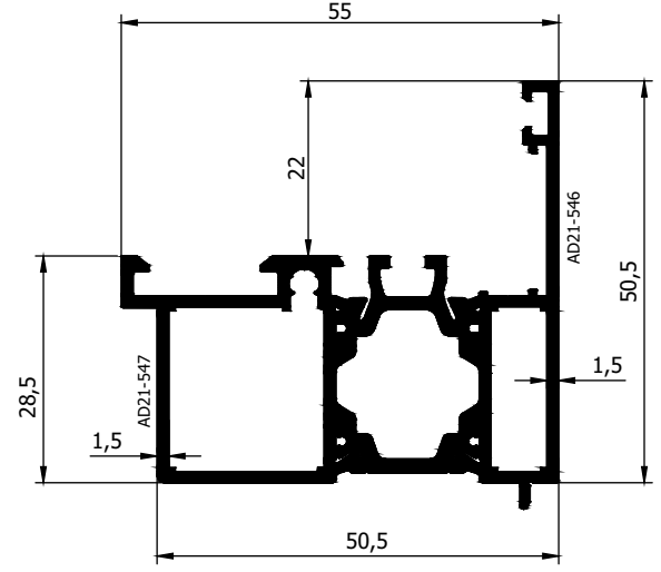
AD 21 - 026 ( 1,135 Kg/m ) Jx : 12,97 cm 4 | Jy : 6,46 cm 4
