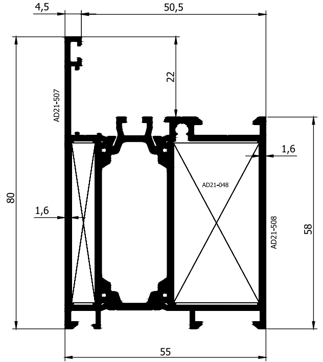
AD 21 - 004 ( 1,685 Kg/m )
