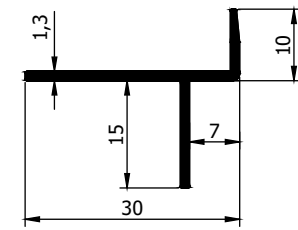
AD 20 - 035 ( 0,186 Kg/m )
