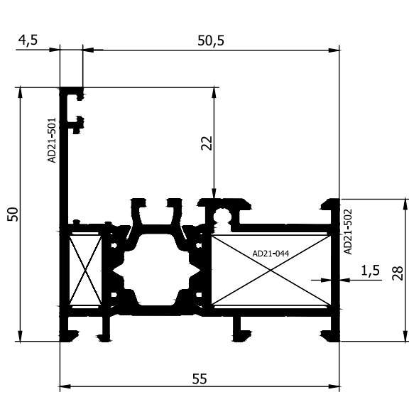
AD 21 - 001 ( 1,148 Kg/m )
