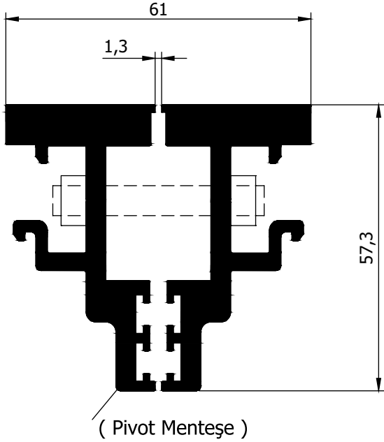
AD 21 - 049 ( 1,575 Kg/m )
