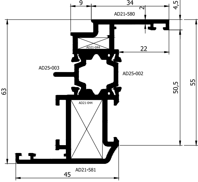
AD 21 - 061 ( 1,500 Kg/m )
