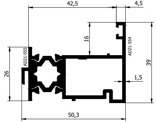
AD 21 - 030 ( 0,930 Kg/m )
