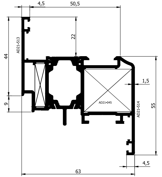
AD 21 - 008 ( 1,435 Kg/m ) Jx : 29,72 cm 4 | Jy : 9,62 cm 4
