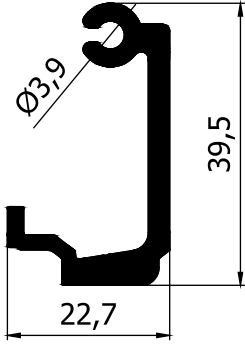
ORTA KAYIT BAĞLANTI PROFİLİ AD21-074 (0,623 Kg/m)
