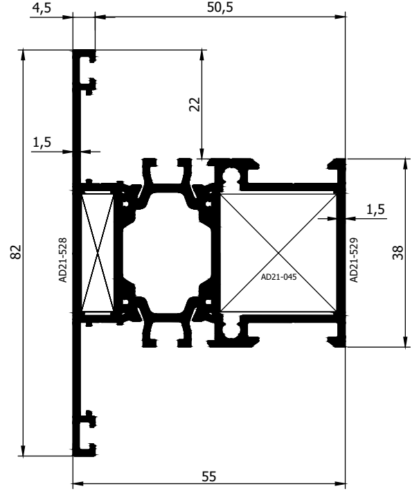
AD 21 - 016 ( 1,460 Kg/m )
