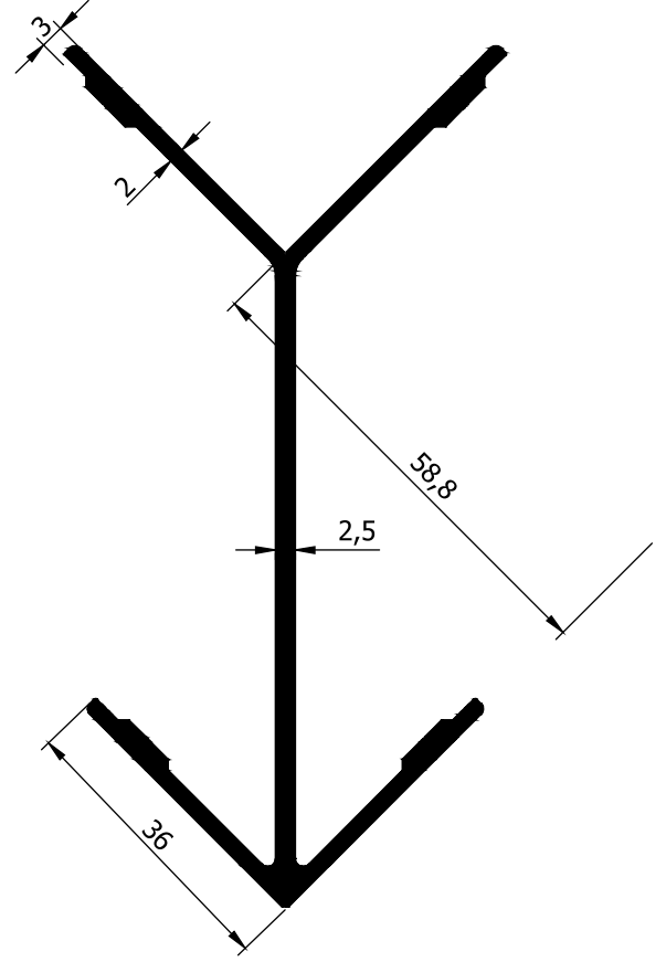
AD 20 - 051 ( 1,415 Kg/m )
