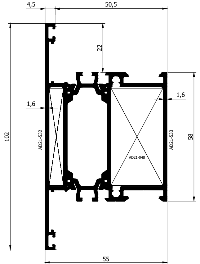
AD 21 - 018 ( 1,835 Kg/m )
