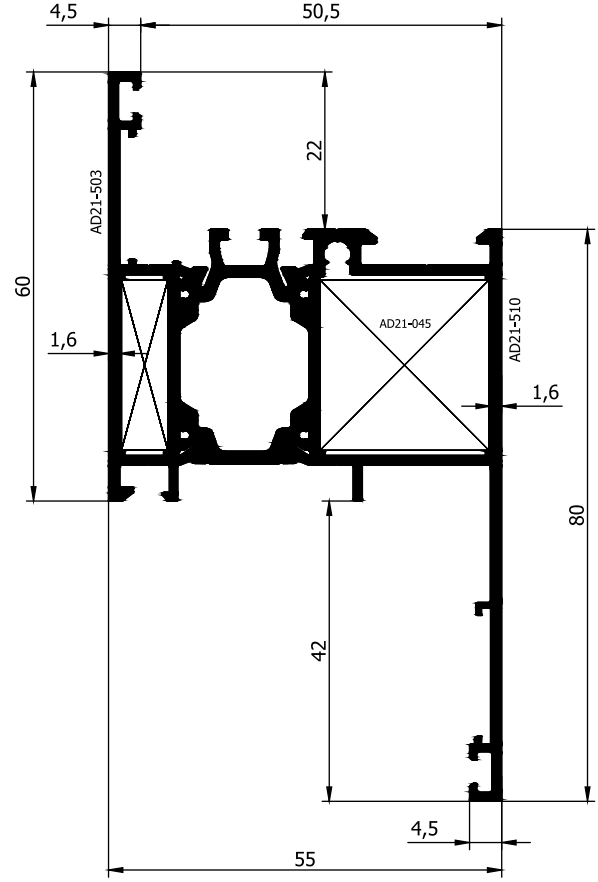
AD 21 - 006 ( 1,530 Kg/m )
