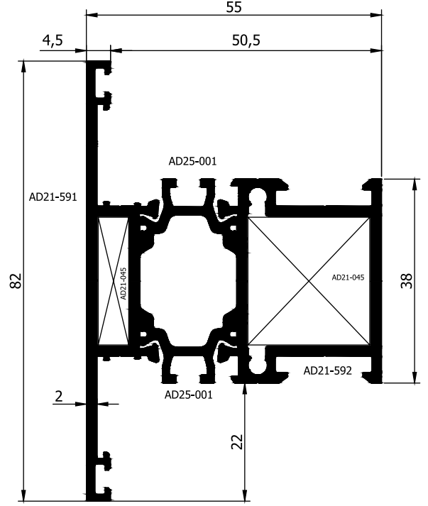
AD 21 - 067 ( 1,724 Kg/m )
