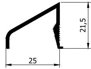
AD 20 - 037 ( 0,228 Kg/m )
