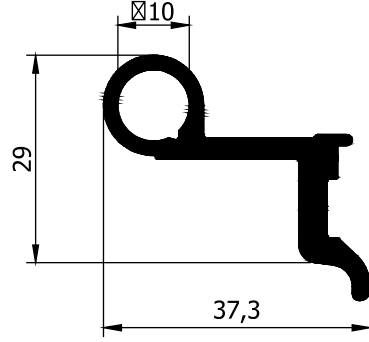
KANAT MENTEŞE AD21-081 (0,640 Kg/m)
