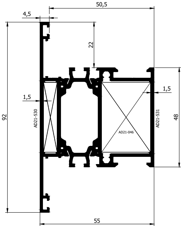
AD 21 - 017 ( 1,620 Kg/m )
