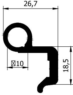
KASA MENTEŞE AD21-080 (0,575 Kg/m)
