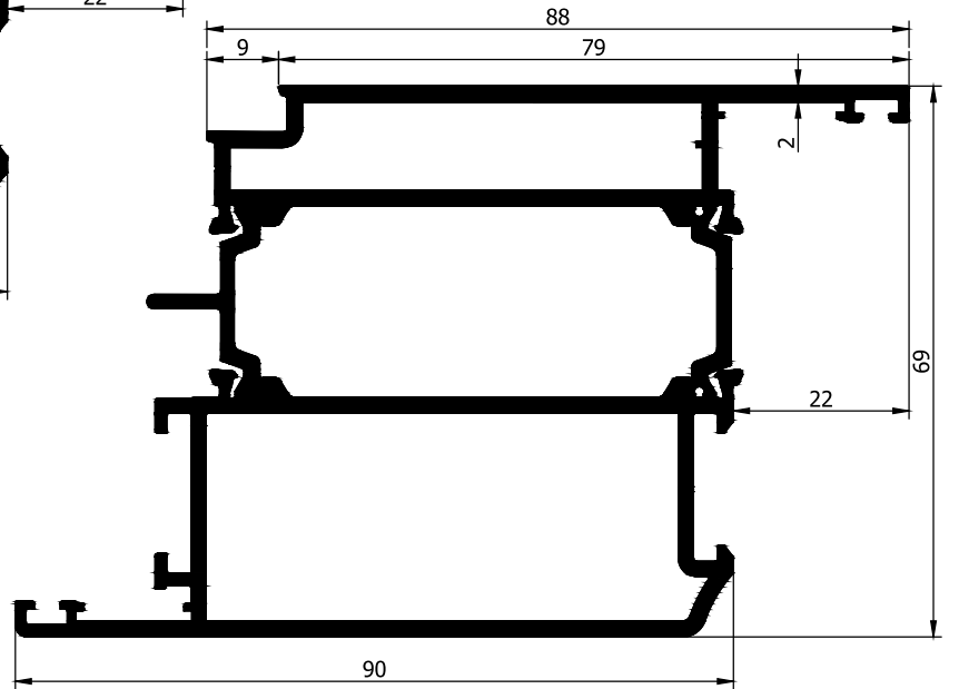
AD31-032 2,485 Kg/m
