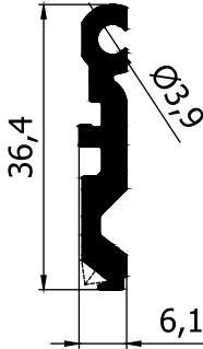
ORTA KAYIT BAĞLANTI PROFİLİ (SETSKURLU)
