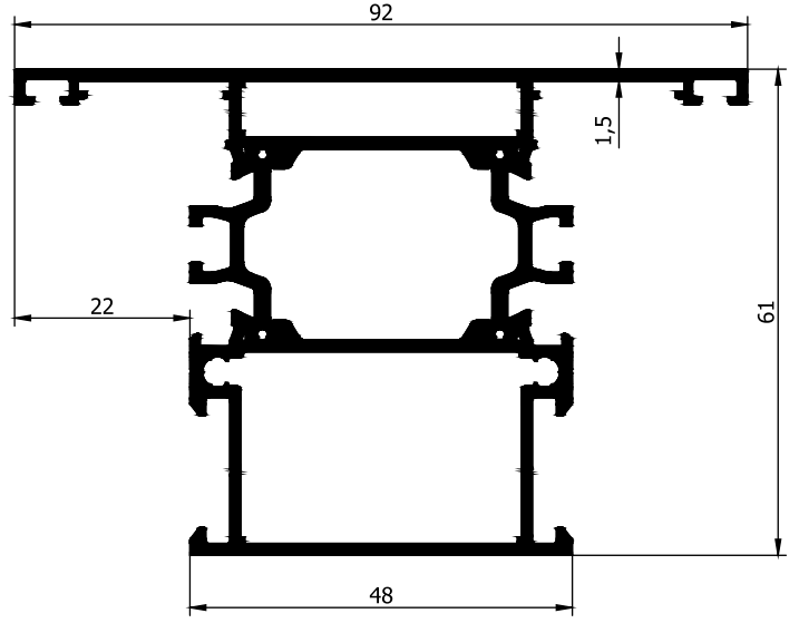
AD31-017 1,671 Kg/m
