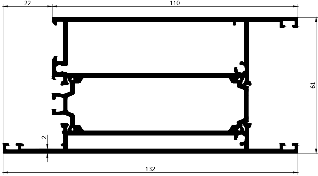
AD31-049 2,954 Kg/m
