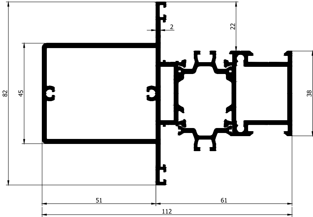
AD31-050 2,617 Kg/m
