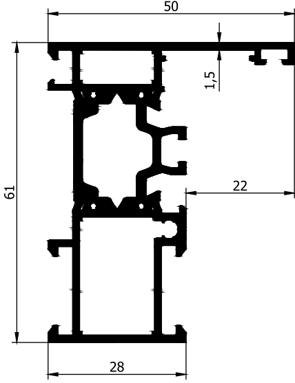
AD31-001 1,193 Kg/m
