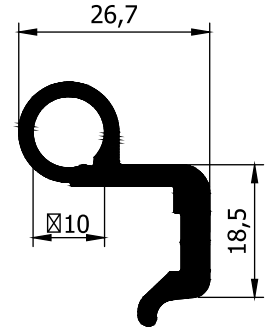
KASA MENTEŞE
