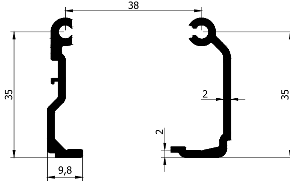
ORTA KAYIT BAĞLANTI PROFİLİ
