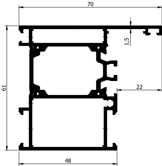
AD31-003 1,518 Kg/m
