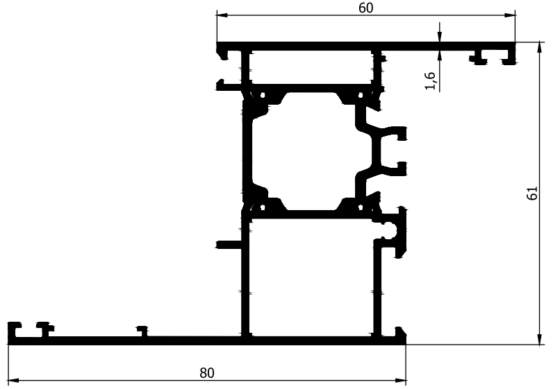
AD31-006 1,573 Kg/m
