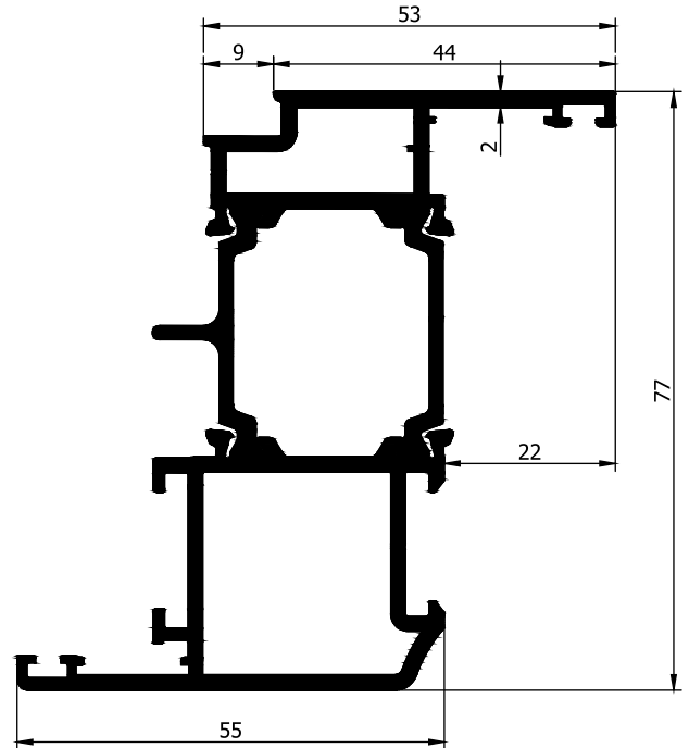
AD32-031 1,784 Kg/m
