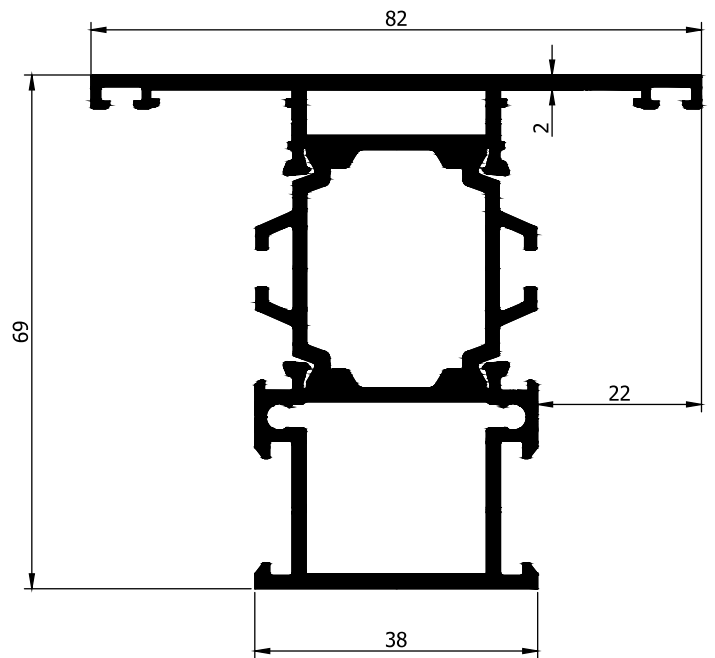
AD32-046 1,818 Kg/m
