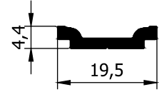
AD20-038 0,130 Kg/m
