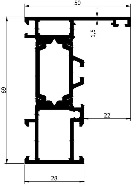
AD32-001 1,234 Kg/m
