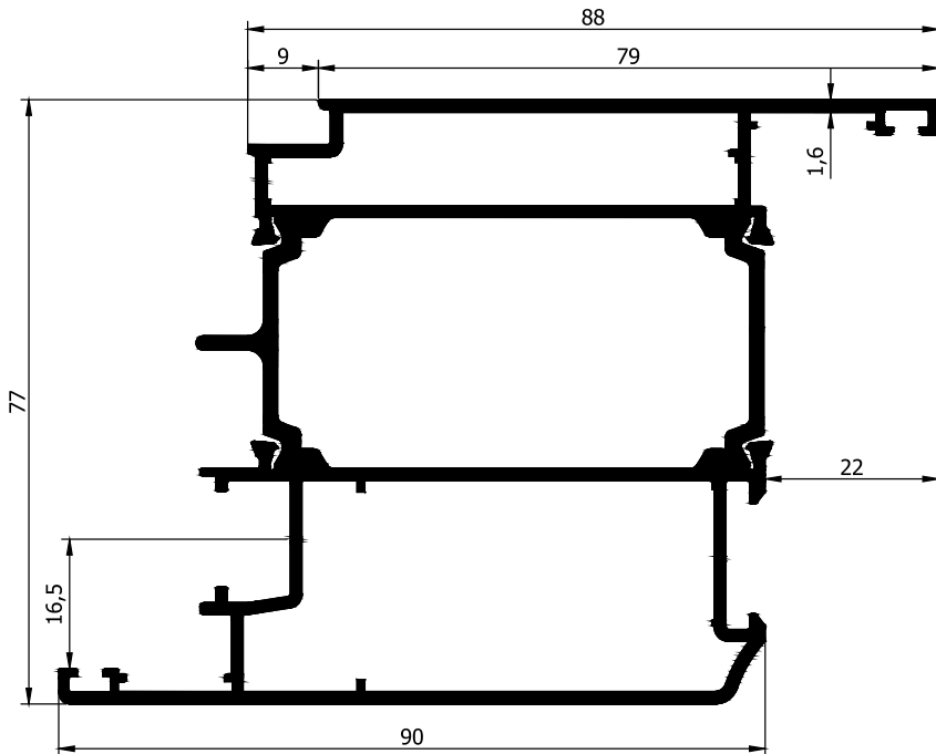
AD32-023 2,154 Kg/m
