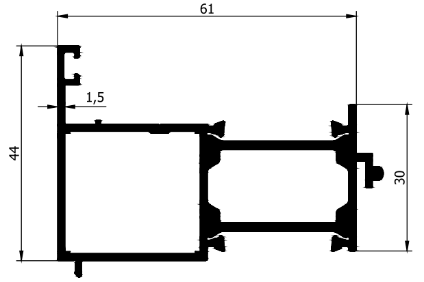
AD32-056 1,039 Kg/m
