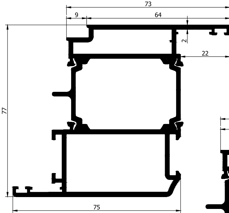
AD32-043 2,206 Kg/m
