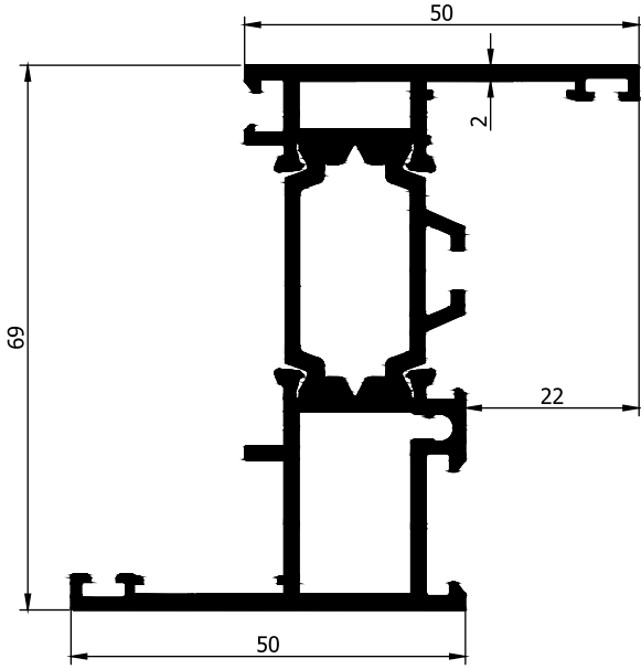
AD32-038 1,558 Kg/m
