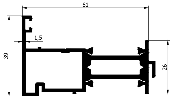
AD32-058 0,976 Kg/m
