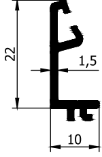
AD 21 - 040 0,179 Kg/m
