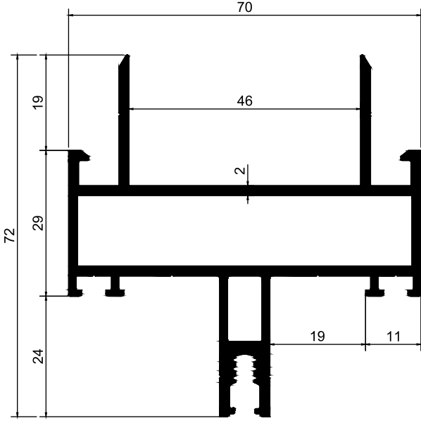
YATAY PROFİL
