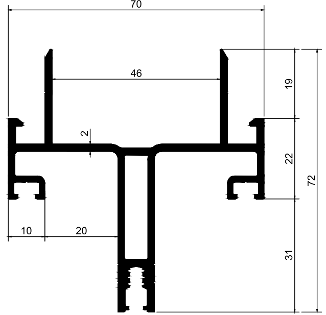
DÜŞEY PROFİL
