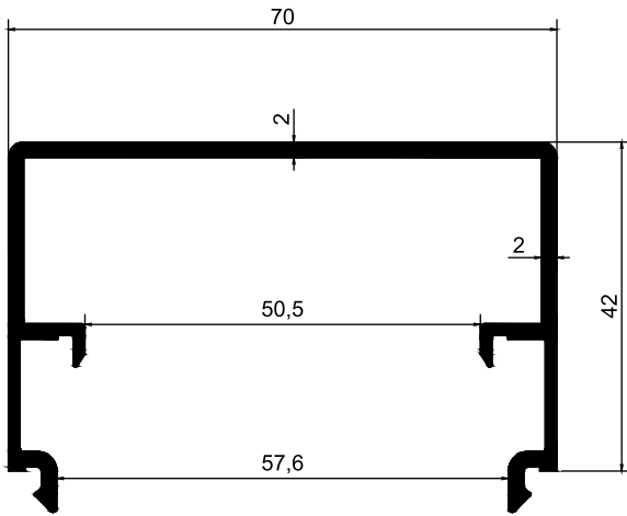
42 LİK KAPAK PROFİLİ
