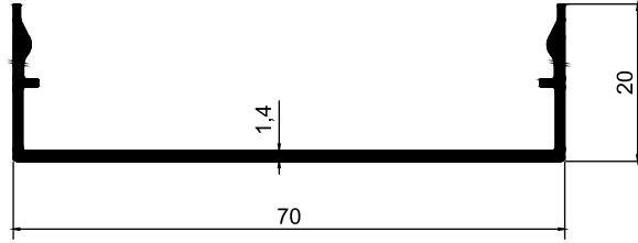
20 LİK BASKI KAPAĞI PROFİLİ AD 29 - 008 ( 0,412 Kg/m )
