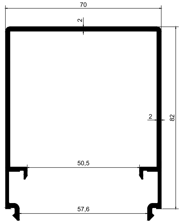
82 LİK KAPAK PROFİLİ
