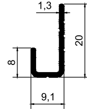
F PROFİLİ AD 07 - 006 ( 0,114 Kg/m )
