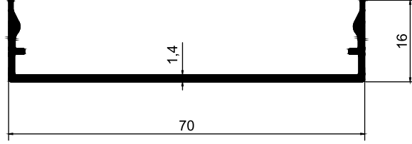
16 LİK BASKI KAPAĞI PROFİLİ AD 29 - 007 ( 0,385 Kg/m )
