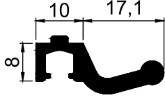
AD 22 - 050 ( 0,327 Kg/m ) 150°
