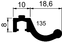
AD 22 - 049 ( 0,350 Kg/m ) 135°
