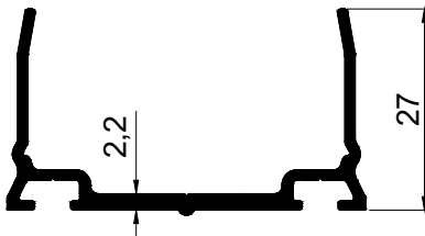
AD 22 - 034 ( 0,488 Kg/m )
