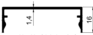
AD 22 - 031 ( 0,312 Kg/m )
