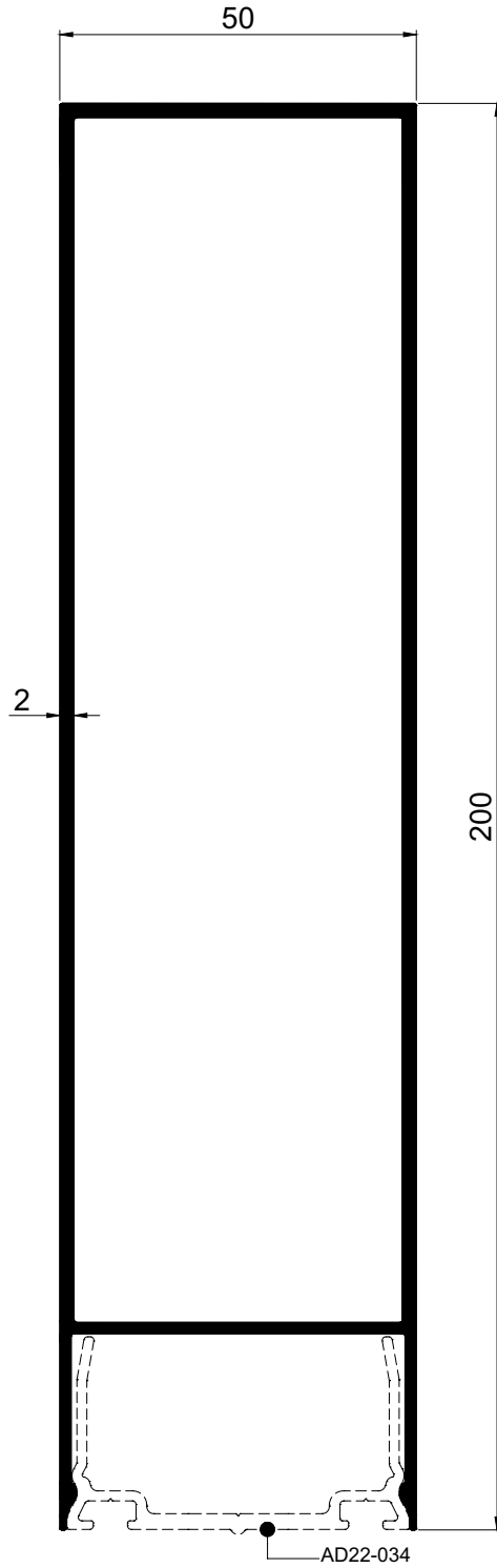
AD 22 - 091 ( 2,556 Kg/m )
