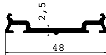
AD 22 - 033 ( 0,408 Kg/m )
