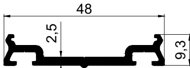
AD 22 - 033 ( 0,408 Kg/m )
