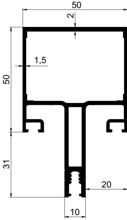
AD 22 - 001 ( 1,535 Kg/m )
