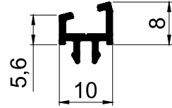
AD 22 - 074 ( 0,106 Kg/m ) 150°
