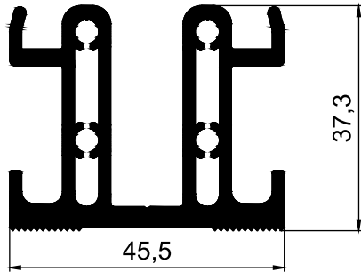
AD 22 - 060 ( 1,582 Kg/m )
