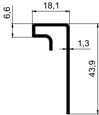
AD 22 - 063 ( 0,273 Kg/m )
