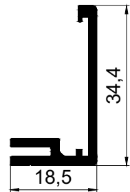
AD 22 - 026 ( 0,340 Kg/m )
