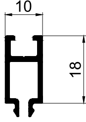
AD 22 - 068 ( 0,196 Kg/m )
