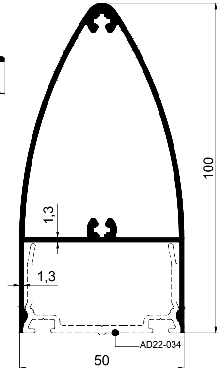
AD 22 - 036 ( 1,182 Kg/m )
