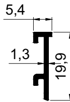
AD 22 - 024 ( 0,108 Kg/m )
