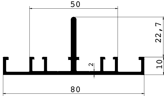
AD 23 - 012 ( 0,890 Kg/m )
