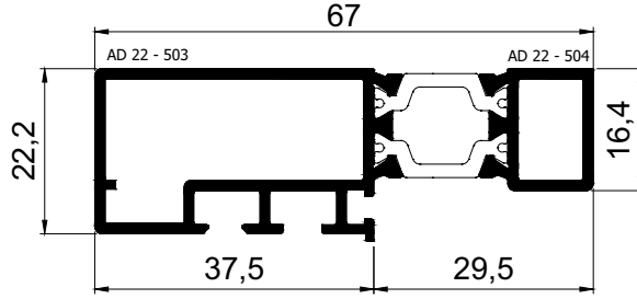
AD 22 - 027 ( 0,942 Kg/m )
