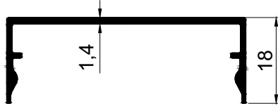
AD 22 - 030 ( 0,325 Kg/m )
