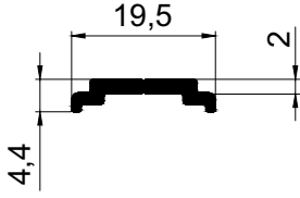
AD 22 - 055 ( 0,120 Kg/m )
