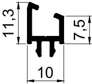
AD 22 - 073 ( 0,124 Kg/m ) 135°
