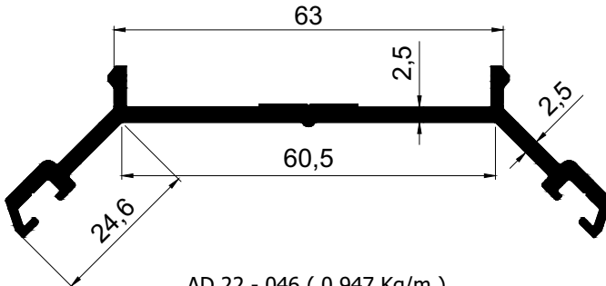
AD 22 - 046 ( 0,947 Kg/m )
