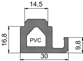
AD 22 - 054 ( 0,290 Kg/m )
