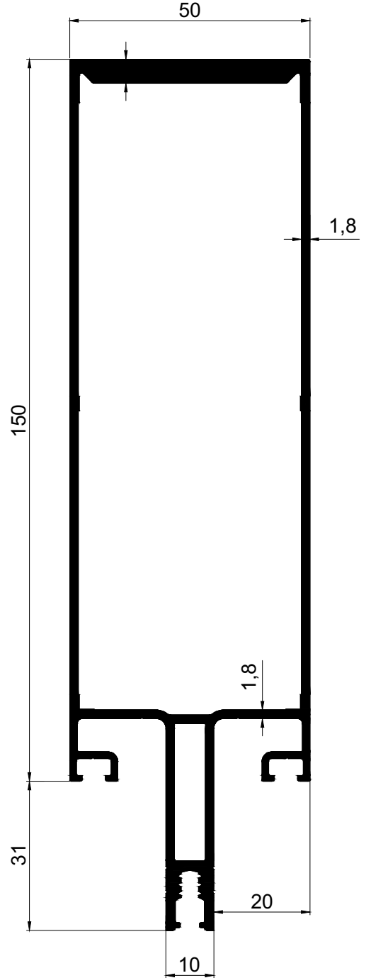
AD 22 - 006 ( 2,915 Kg/m )
