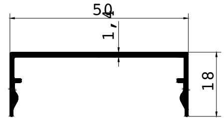
AD 22 - 030 ( 0,325 Kg/m )
