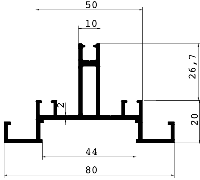
AD 23 - 011 ( 1,145 Kg/m )
