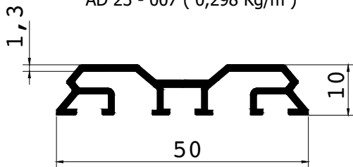
AD 23 - 008 ( 0,383 Kg/m )
