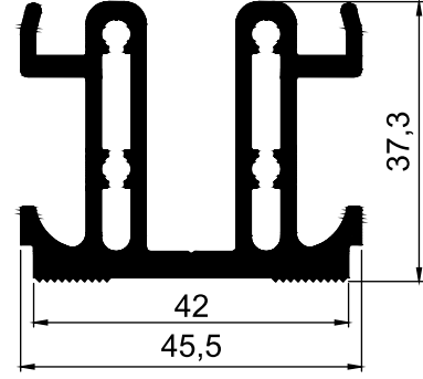
AD 22 - 079 ( 1,547 Kg/m )
