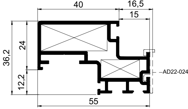
AD 22 - 018 ( 0,843Kg/m )
