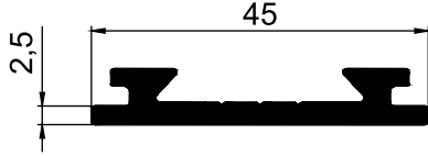
AD 22 - 057 ( 0,501 Kg/m )
