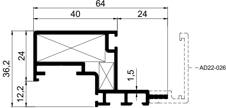
AD 22 - 025 ( 0,805 Kg/m )
